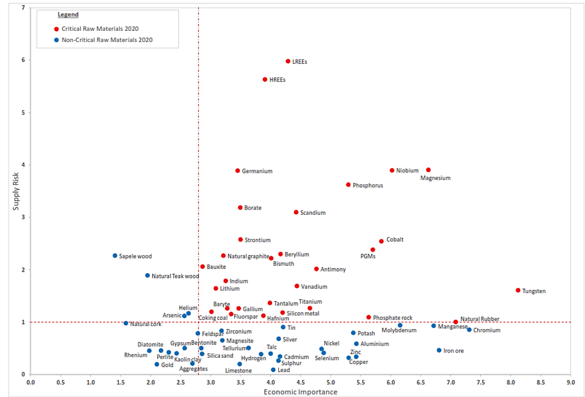
Kuva 3. Kriittisyyden arviointien kokonaistulokset, jotka on kartoitettu kriittisyydskynnyksiin. Kriittiset raaka-aineet on korostettu punaisilla pisteillä ja ne sijaitsevat kriittisyydsvyöhykkeellä ( SR \geq 1 ja EI \geq 2,8 ). Siniset pisteet edustavat ei-kriittisiä raaka-aineita 7 .
