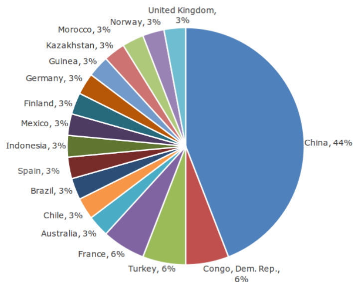
Kuva 8. Tärkeimmät EU:n kriittisten raaka-aineiden hankintamaat (perustuu toimitettujen raaka-aineiden lukumäärään), keskiarvo vuosilta 2012–2016 (REE osalta 2016–2018) 12 .
